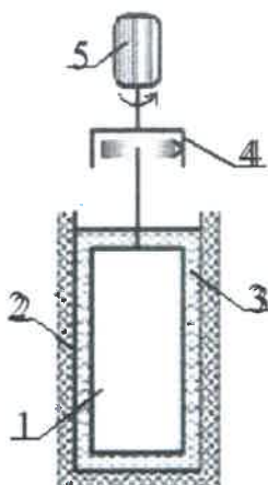
Рисунок 1 - Принципиальная схема ротационного вискозиметра 1 - шпindelь, 2 - сосуд, 3 - проба вязущего; 4 - измерительный механизм, 5 – двигатель
