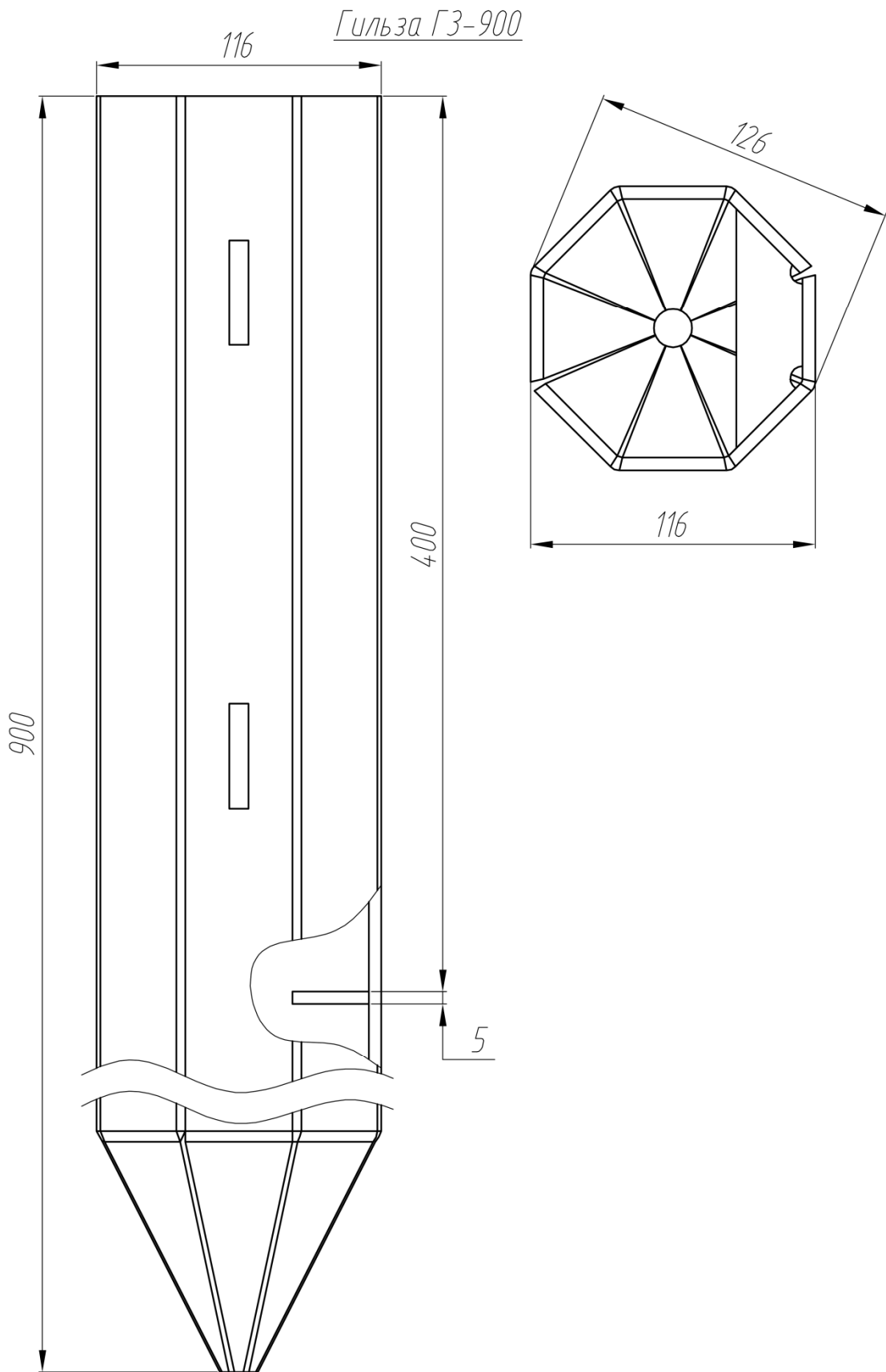
Рисунок А.9 – Гильза ГЗ-900
