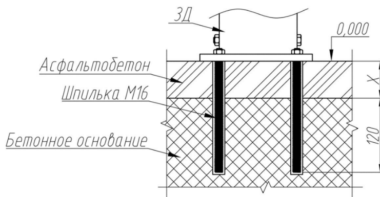
Рисунок 9.2 – Схема установки закладной детали ЗД
