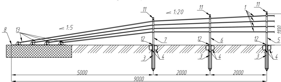
Начальный (концевой) участок марки 23ДО(ДД)-Н(К)/С-1,1-2,0-9,0-ГЗГ
