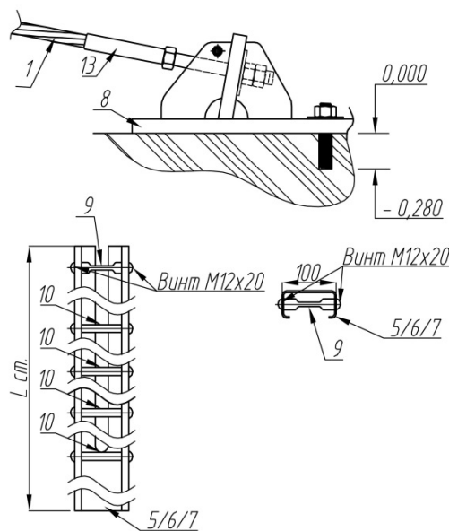
Рисунок А.2 - Схема и состав ограждений марки 23ДО(ДД)-Н(К)/С-1,1-2,0-9,0
