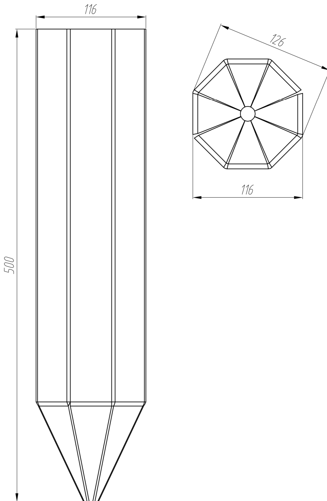
Гильза ГЗ-500
