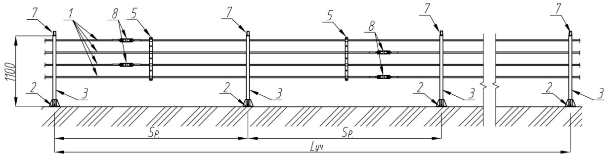
Рабочий участок мостового ограждения марки 23МД/У4-П-Н-Ср-у (В)
