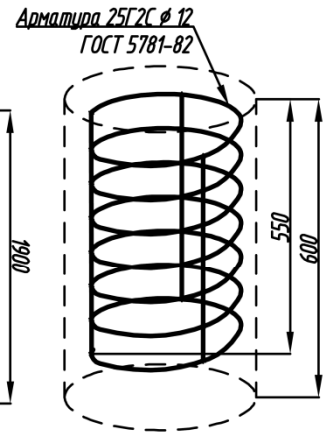
Схема армирования фундамента гильзы (заводское изготовление)
