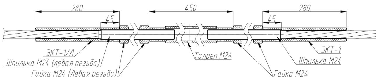
Рисунок 9.4 – Талреп в сборе
