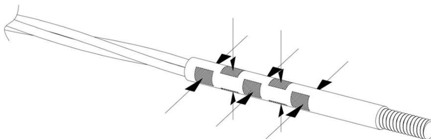
Рисунок 9.3 – Схема обжатия троса элементом концевым
