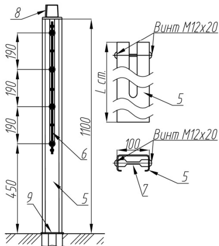
Рисунок А.1- Схема и состав ограждений марки 23ДД(ДО)/УЗ(У4)-С-1,1-Ср-у(В)
