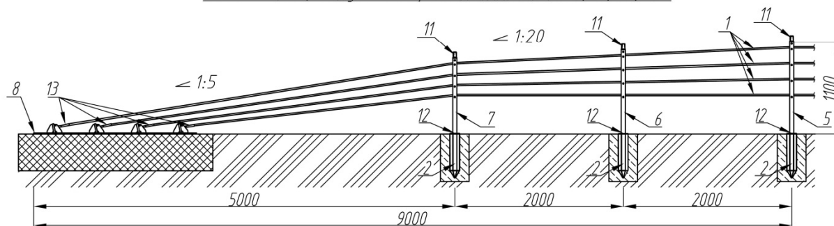
Начальный (концевой) участок марки 23ДО(ДД)-Н(К)/С-1,1-2,0-9,0-ГБ
