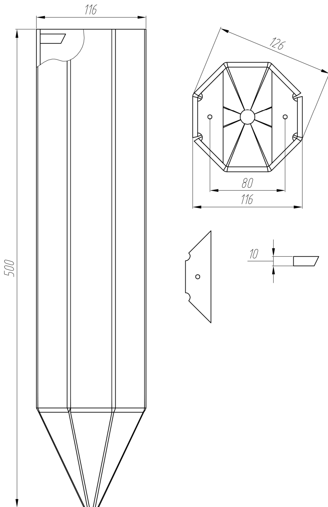
Гильза ГЗ-500/У
