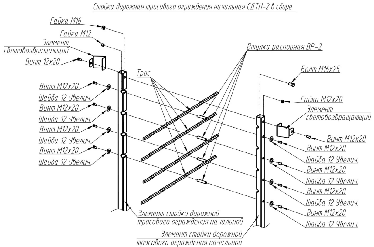
Рисунок А.7 - Схема монтажа ограждений
