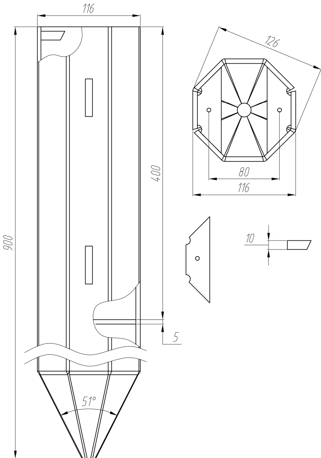
Гильза ГЗ-900/У
