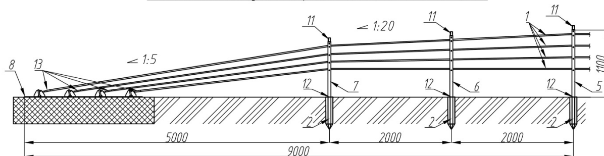
Начальный (концевой) участок марки 23ДО(ДД)-Н(К)/С-1,1-2,0-9,0-ГЗ
