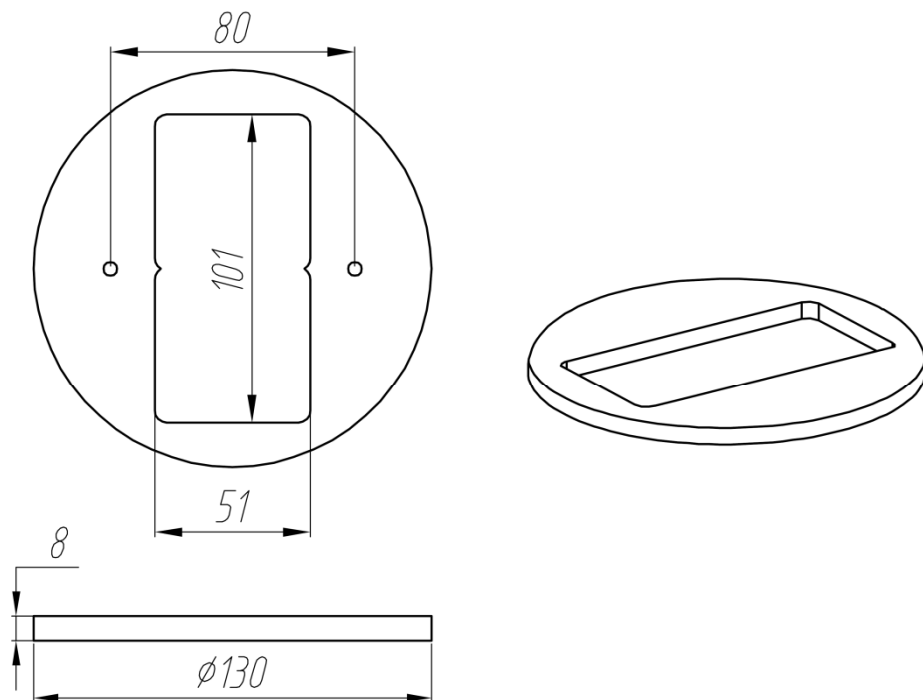
Заглушка гильзы ЗГ-2
