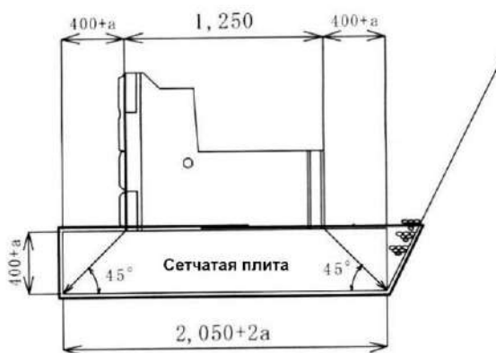
Рисунок 6 - Схема устройства габионно-сетчатой плиты (матрац Рено).
