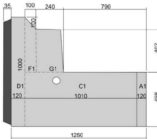
Рисунок А.2. - Блок конструктивный железобетонный КБП 100/150
