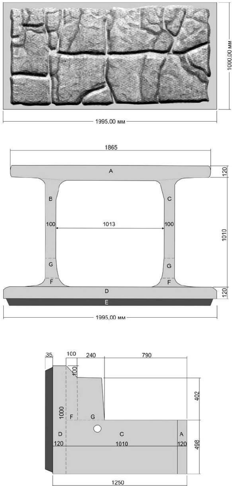
Рисунок А.1. - Блок конструктивный железобетонный КБП 100/200
