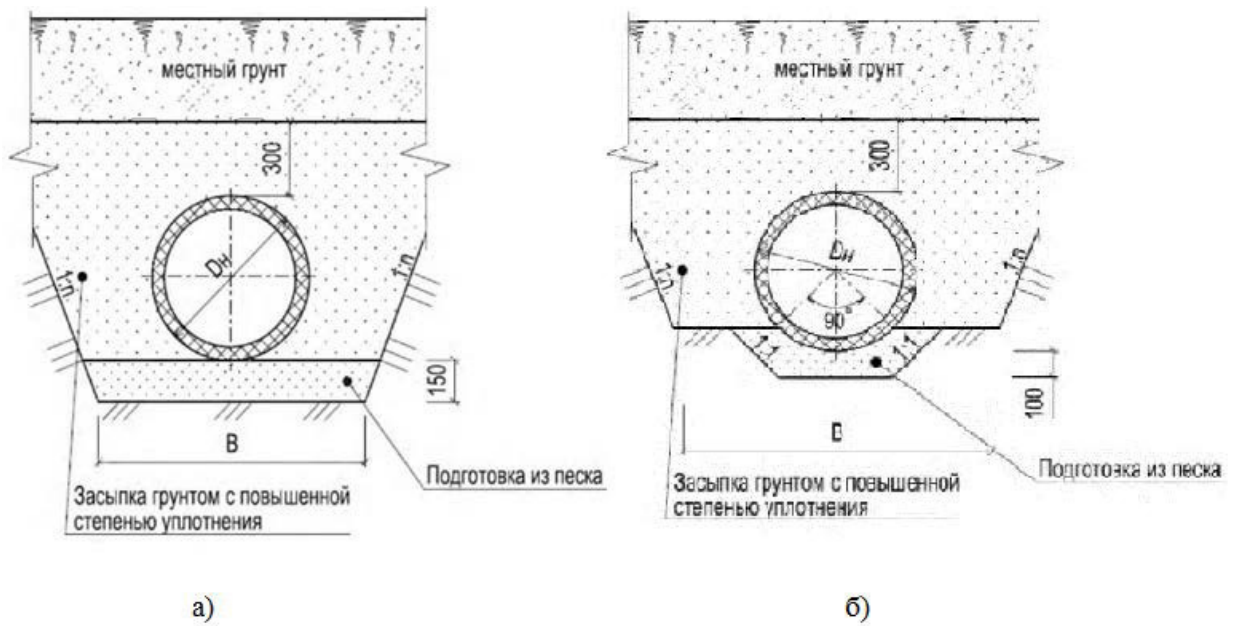
Рисунок 9 – Схема укладки труб, грунт основания: глинистые, гравелистые грунты, крупнообломочные скальные породы
