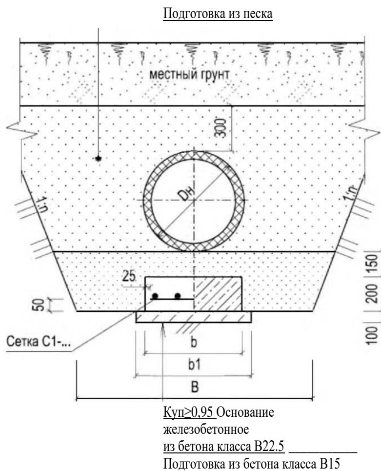
Рисунок 11 – Схема укладки труб, грунт основания: грунты с возможной неравномерной осадкой
