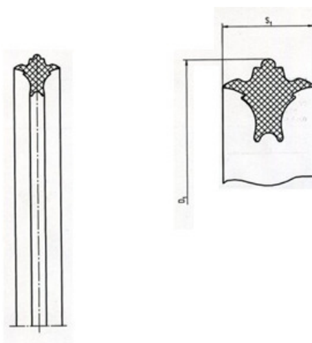
Рисунок 4 – Профиль резинового кольца
