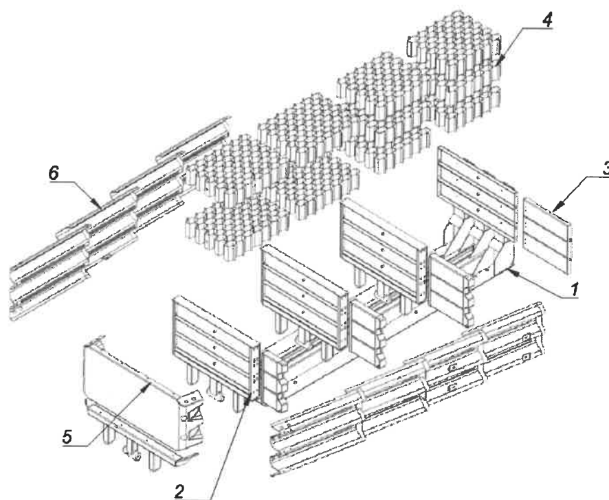
1 - основание, 2 – подвижная рама (диафрагма), 3 – дополнительная панель к подвижной раме (только в не параллельных и ассиметричных системах), 4 - сотовый энергопоглощающий элемент, 5 – бампер, 6 – подвижная боковая панель, Рисунок 1 - Конструкция фронтального ограждения секционного типа
