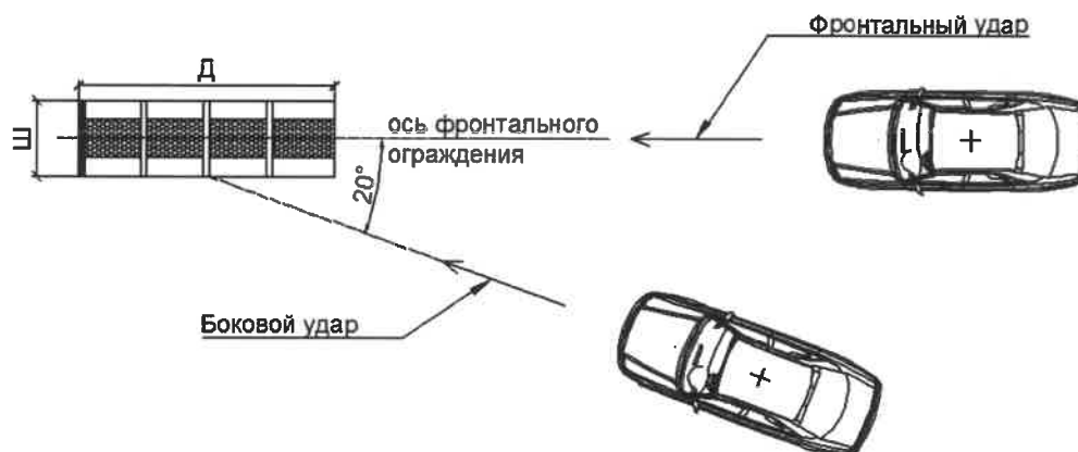
Рисунок Б.1 - Схема натуральных испытаний фронтального ограждения
