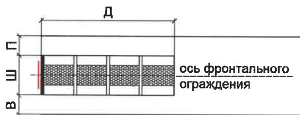
В – деформация ФО со стороны удара, П – деформация фронтального ограждения со стороны противоположной удару
