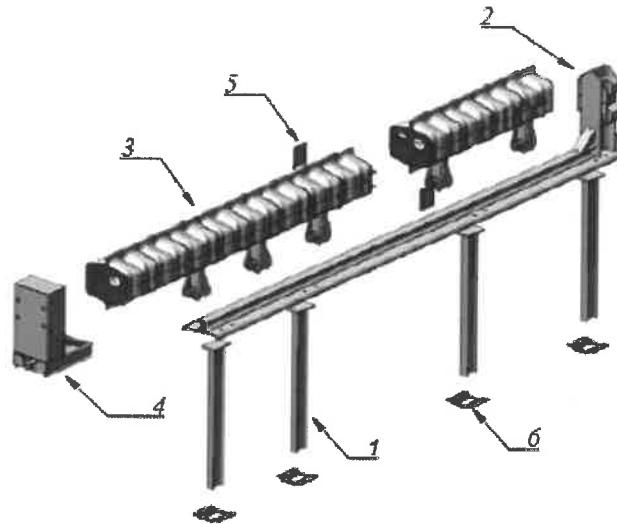
1- Забивная стойка, 2 – основание, 3 – модульный энергопоглощающий элемент, 4 – бампер, 5 – пластины для скрепления энергопоглощающих элементов, 6 – монтажные пластины для крепления основания к земле
