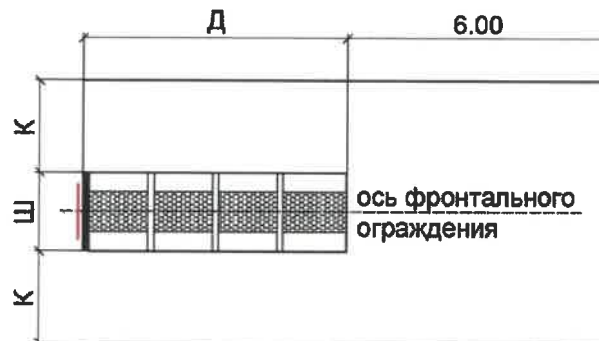
Ш – ширина ограждения, Д – длина ограждения, К – полоса К по ГОСТ 33129 Рисунок Б.2 – Границы коридора выбега ТС после наезда на ограждение
