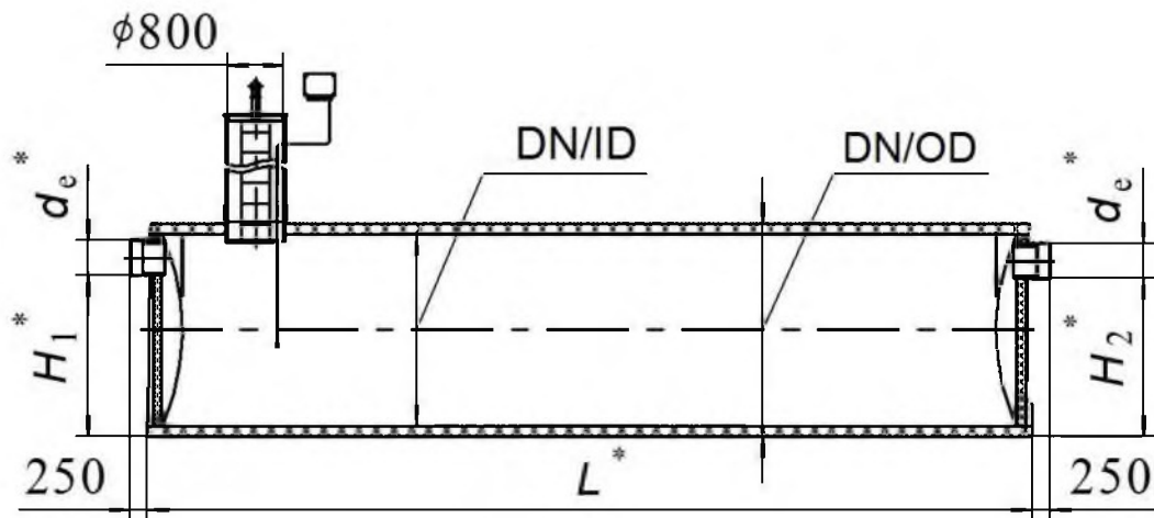
Рисунок 9 – Пескоотделитель (ПЕО)
