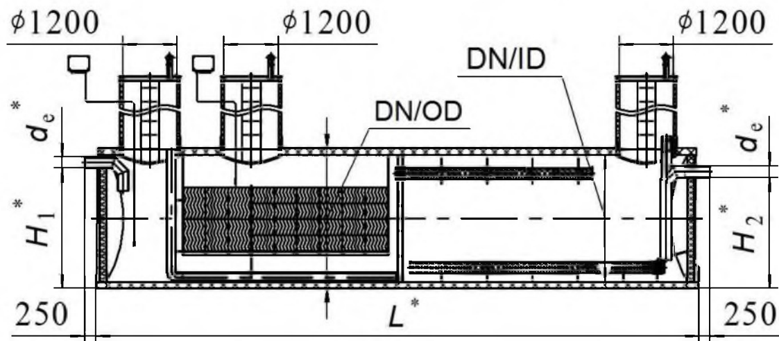
Рисунок 8 – Модифицированное очистное сооружение поверхностного стока (ПЕО-М/МБО/СОФ)
