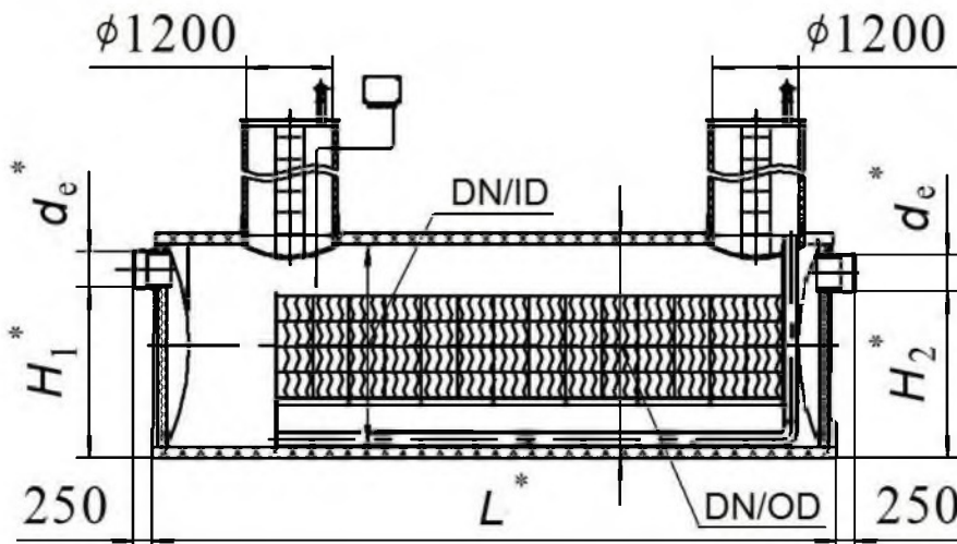
Рисунок 11 – Маслобензоотделитель (МБО)
