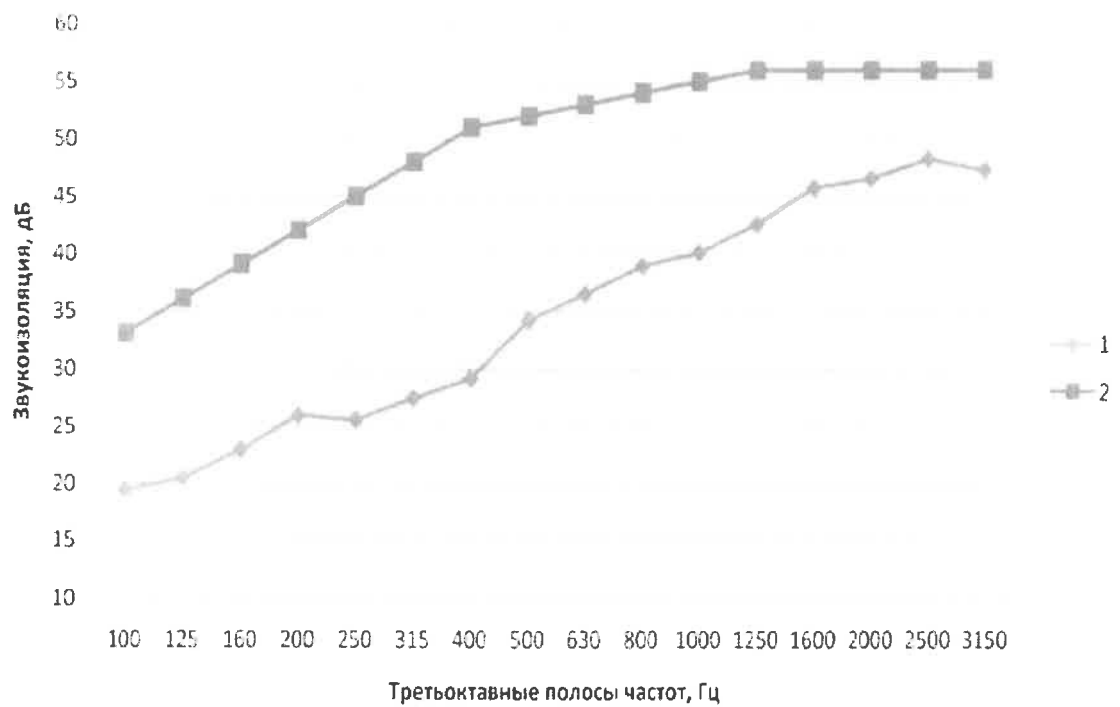
Рисунок 1. Частотные характеристики.
