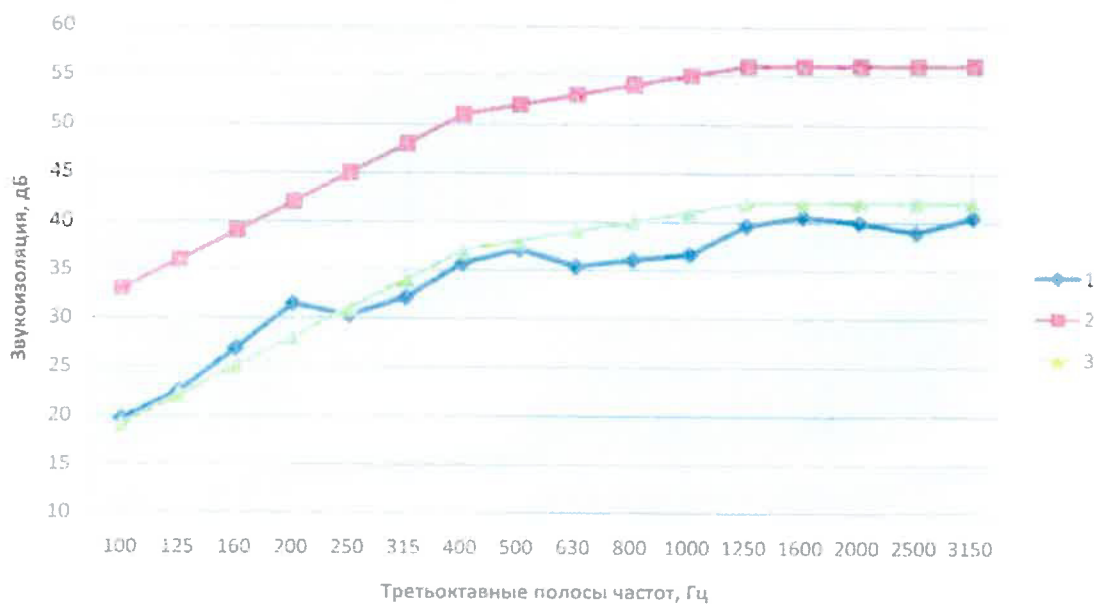
Рисунок 1. Частотные характеристики.
