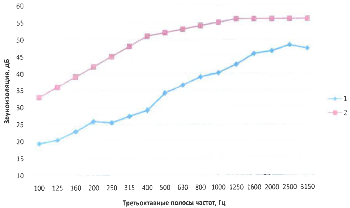
Рисунок 1. Частотные характеристики.
