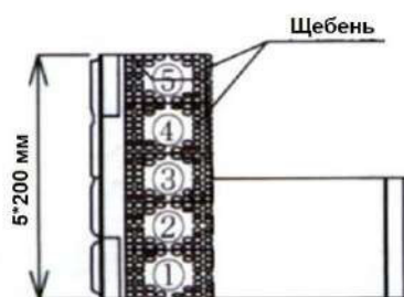
Рисунок 24 - Схема уплотнения щебня у торца.
