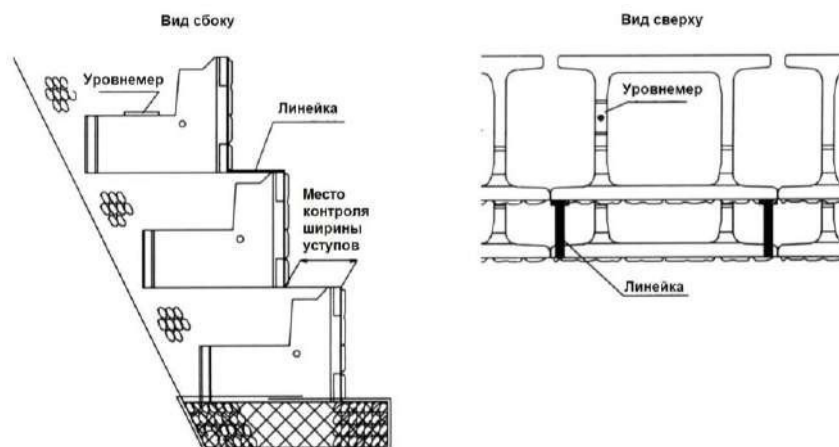
Рисунок 28 - Места контроля ширины уступов.
