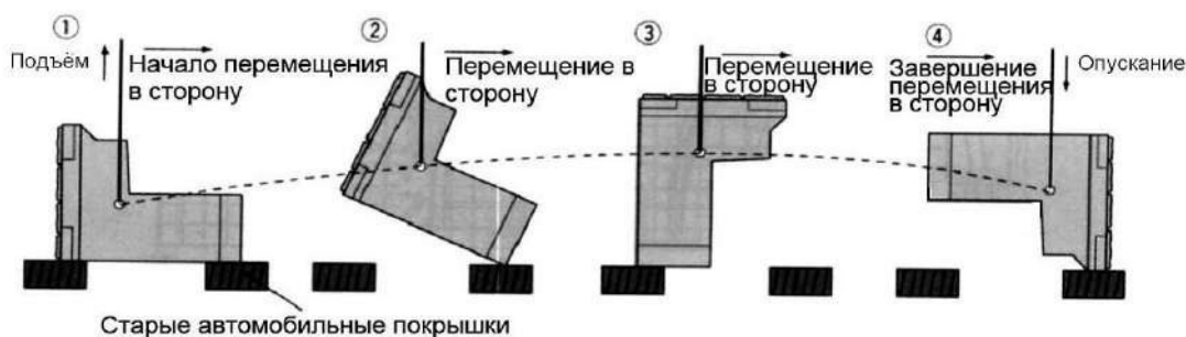
Рисунок 10 - Схема переворачивания блока
