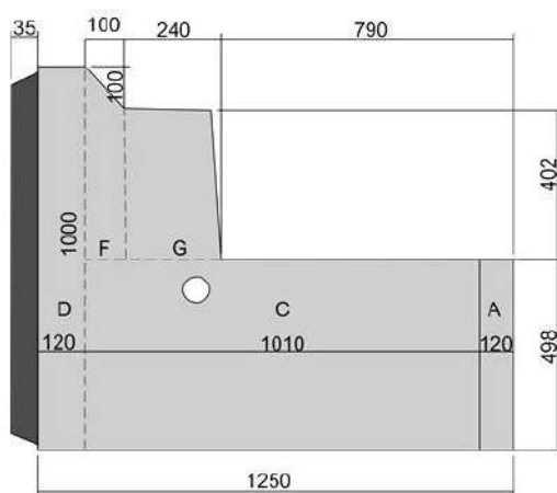
Рисунок А.1. - Блок конструктивный железобетонный КБП 100/200
