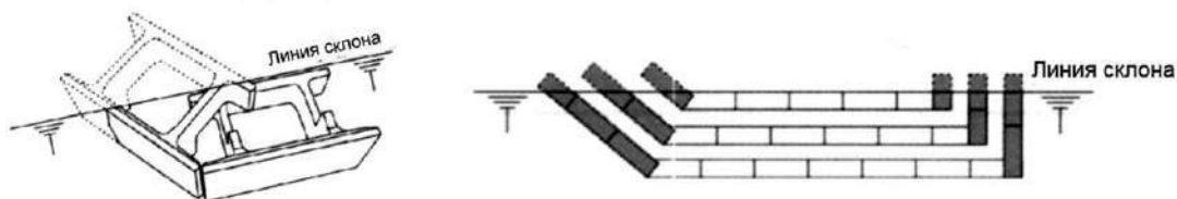
Рисунок 26 - Варианты заделки торцов стены.
