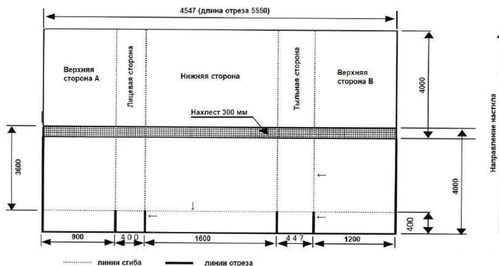
Рисунок 5 - Схема обработки краев стяжной сетки (для уклона 1:0,5).
