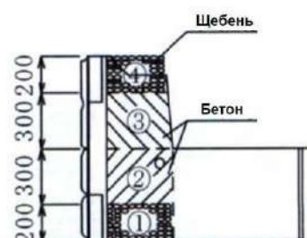
Рисунок 25 - Схема заполнения бетоном и щебнем
