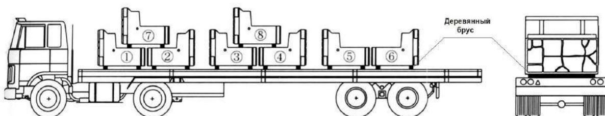
Рисунок 7 - Пример загрузки автомобиля грузоподъемностью 10 т (блоки КБП 200/100).
