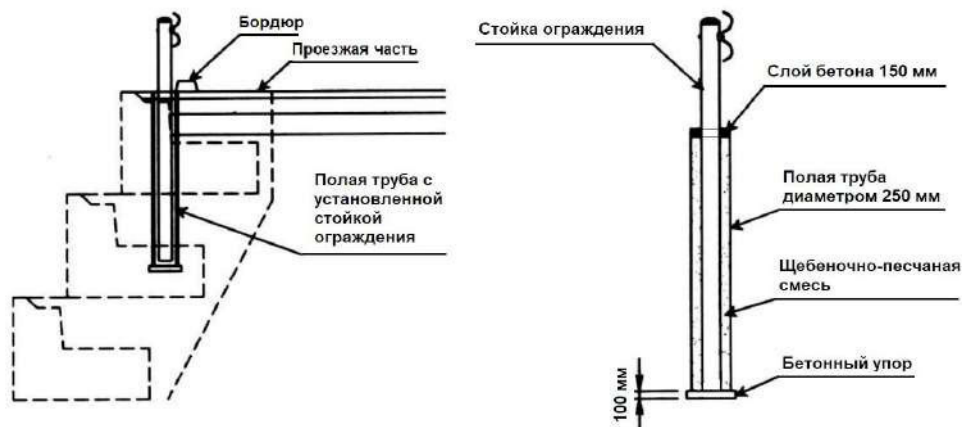
Рисунок 44 - Установка стоек ограждения.
