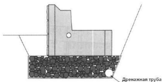
Рисунок 33 - Пример установки водопропускной трубы с желобом.
