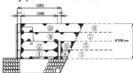
Рисунок 19 - Порядок уплотнения щебня для внутренней засыпки в короба и позади них у подпорной стены для насыпи, а также уплотнения самой насыпи
