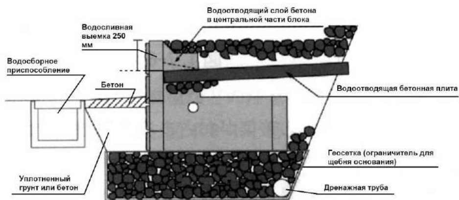
Рисунок 35 - Вариант водоотведения (вид в разрезе).
