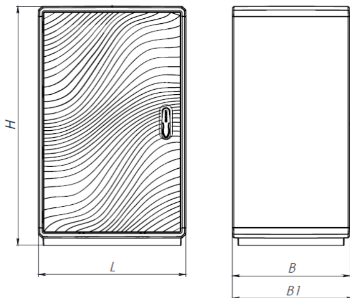
Рисунок А.3 – Эскиз корпуса
