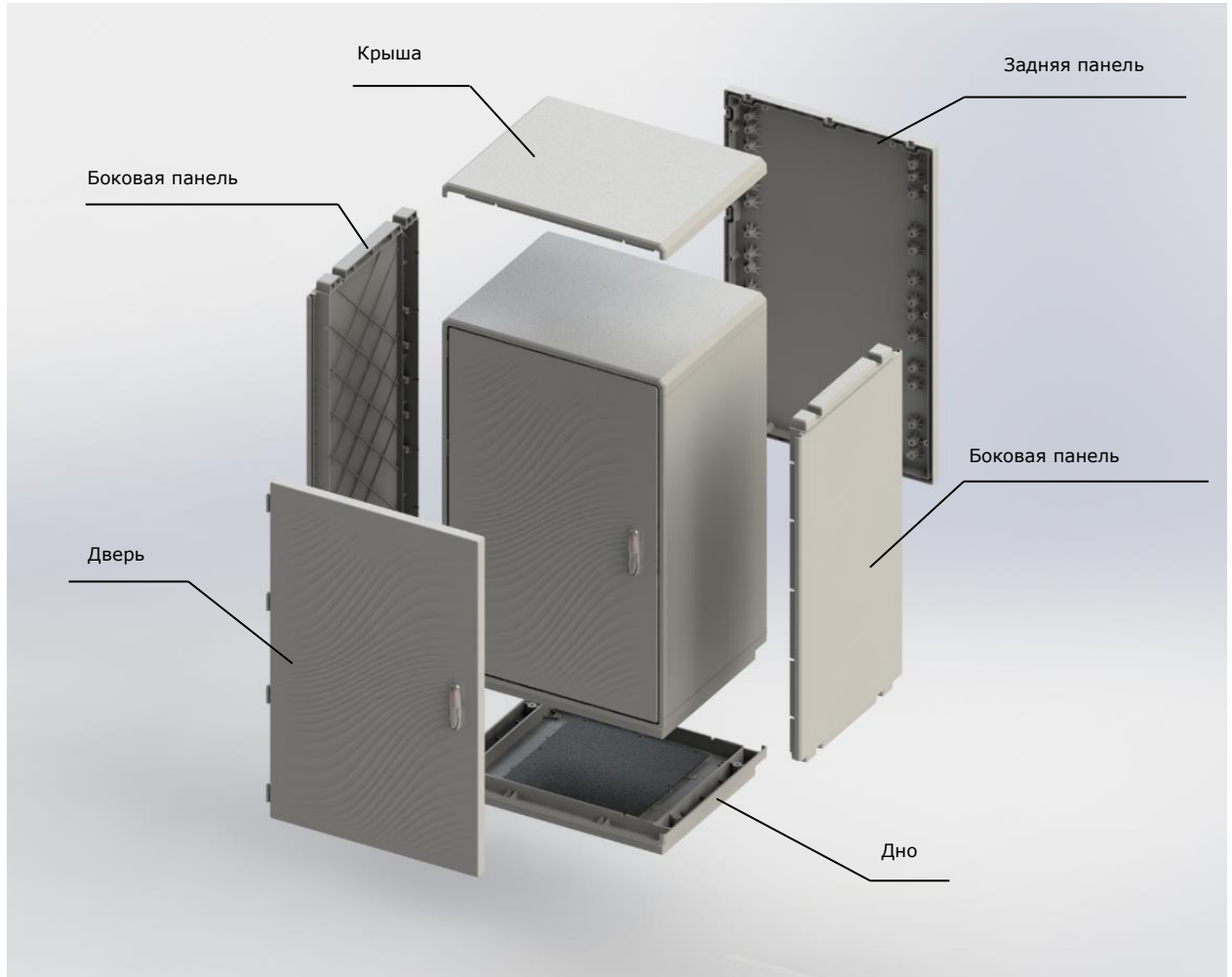
Рисунок А.1 – Составляющие корпуса
