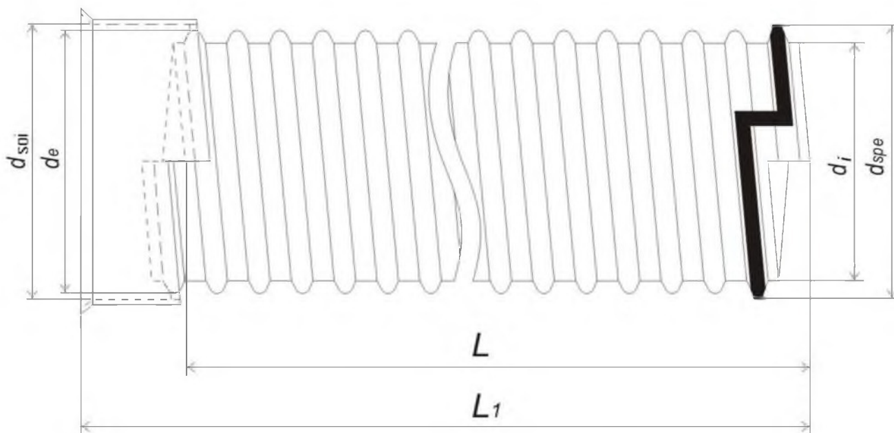
Рисунок 3 – Конструкция труб с раструбным соединением с помощью уплотнительного кольца
