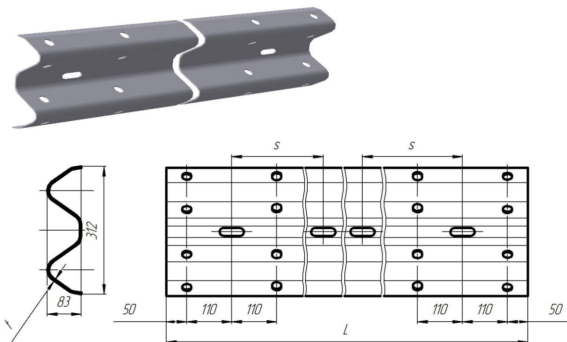
Рисунок Е.5 – Основные параметры секций балок (СБ)
