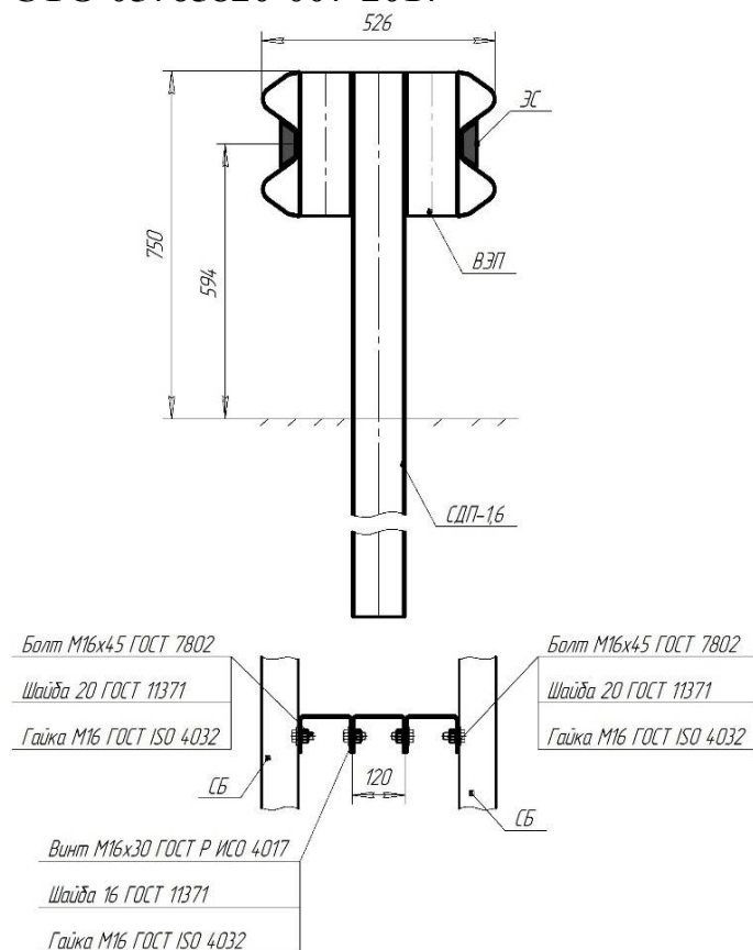
Рисунок В.15 – Ограждение дорожное двустороннее высотой 0,75 м, с применением дорожной стойки СДП-1,6
