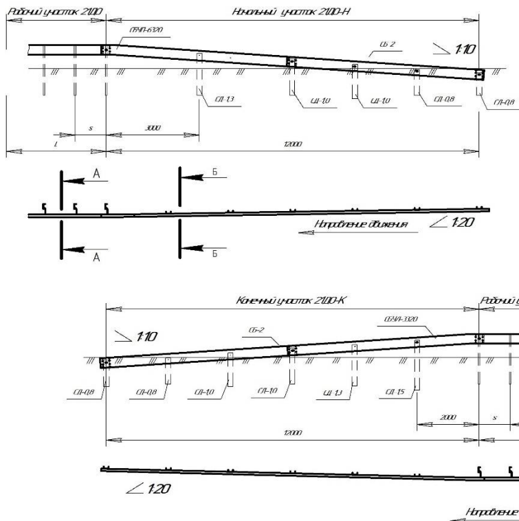
Рисунок И.11 – Схемы монтажа начального (конечного) участков ограждения высотой 0,75 м для дорог IV-ой и V-ой категории с шагом стоек рабочего участка 2,5 м и 3,0 м
