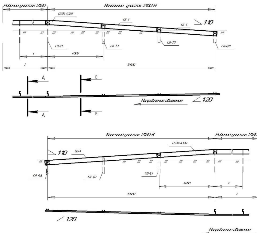
Рисунок И.12 – Схемы монтажа начального (конечного) участков ограждения высотой 0,75 м для дорог IV-ой и V-ой категории с шагом стоек рабочего участка 4,0 м
