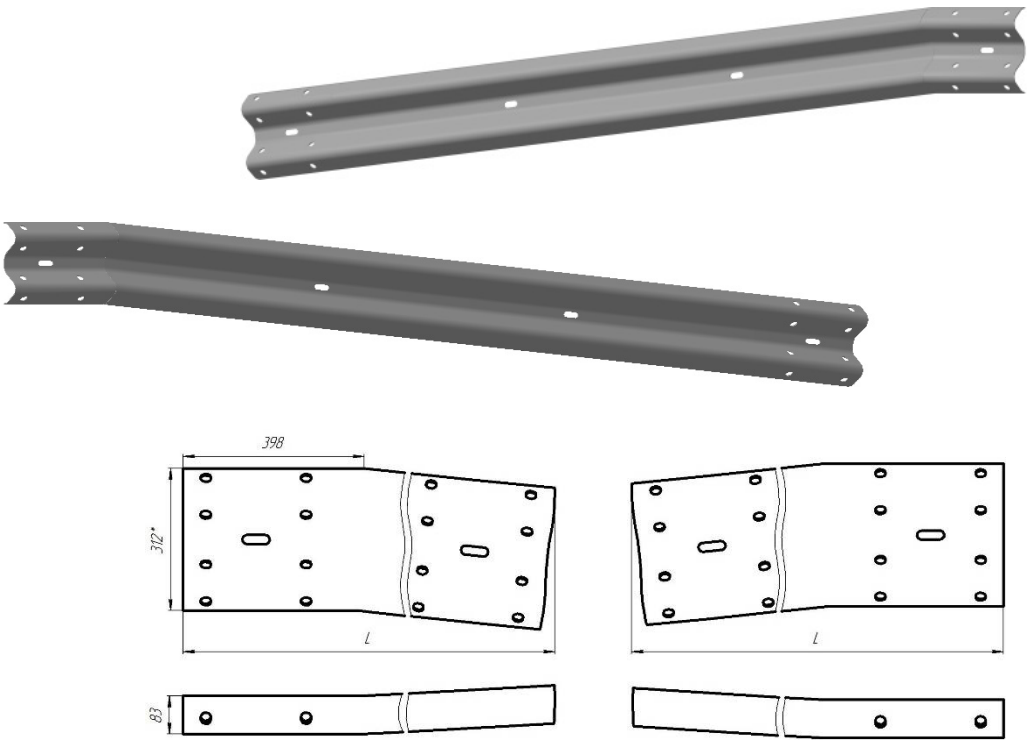
Секция балки угловая правая СБУП Секция балки угловая левая СБУЛ
