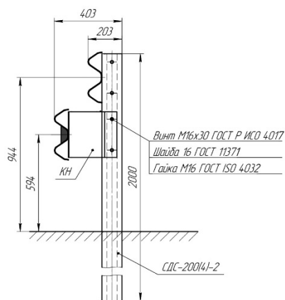
Рисунок В.29.2 – Ограждение дорожное высотой 1,1 м, с применением дорожной стойки СДП(140)-2,0(5,0)-2 без КВ
