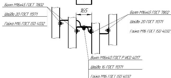
Рисунок В.44.1 – Ограждение дорожное двустороннее высотой 1,1 м с применением дорожной стойки СДС-2,0-3 без КВ
