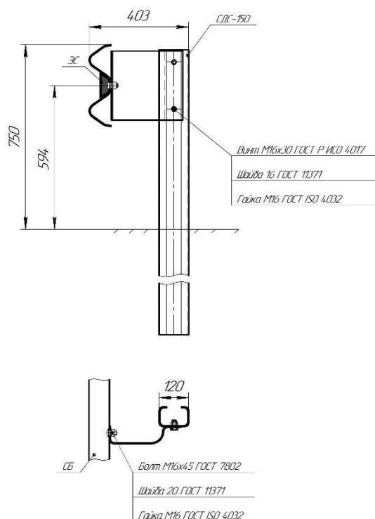
Рисунок В.10 – Ограждение дорожное высотой 0,75 м, с применением дорожной стойки СДС-150
