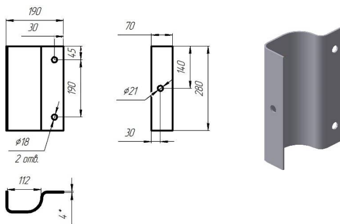
Рисунок Е.3 – Консоль-амортизатор верхний (КВ)
