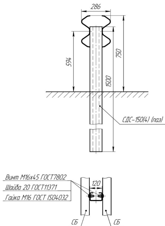
Рисунок В.22.2 – Ограждение дорожное двустороннее высотой 0,75 м, с применением дорожной стойки СДС-150 (паз)
